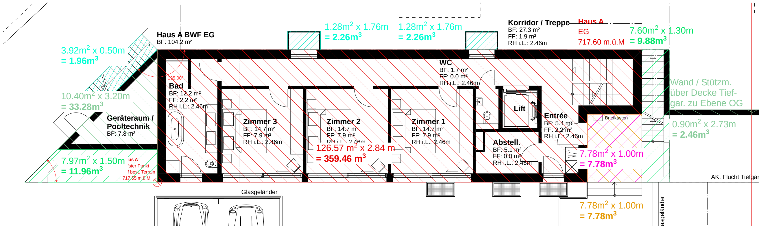
Erdgeschoss
