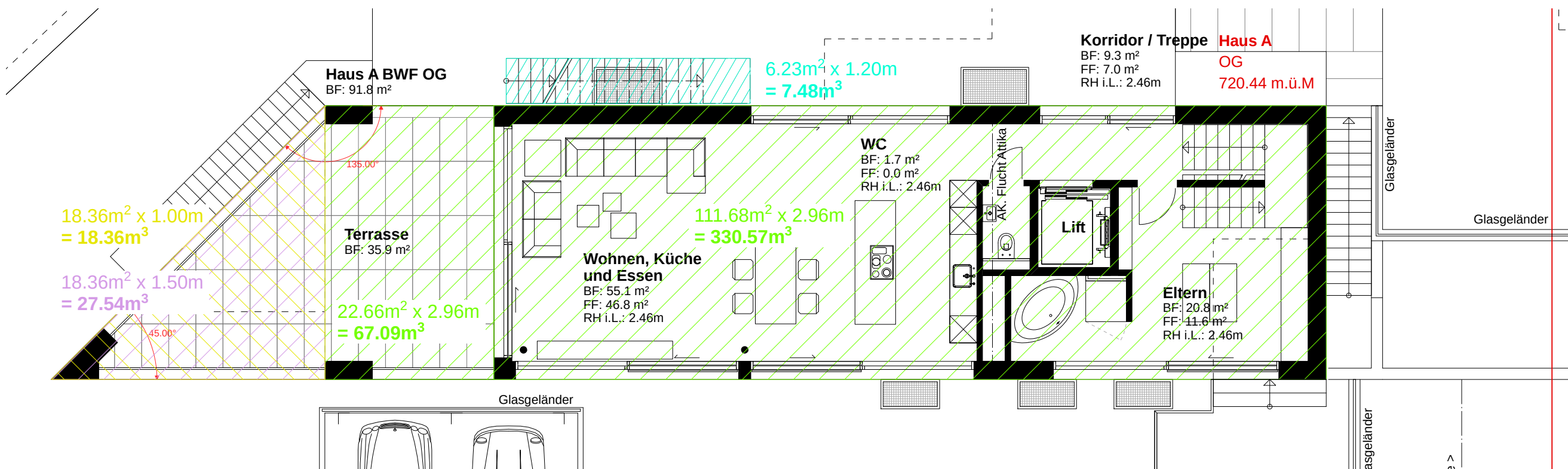
Obergeschoss
